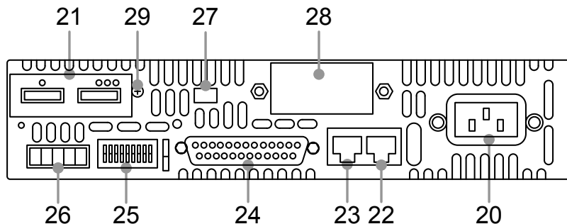
図 3-2 リアパネル
