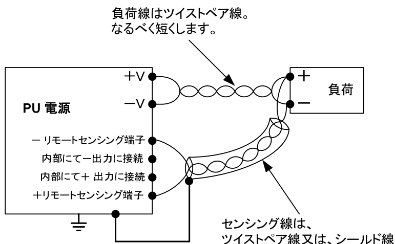
図 2-8 リモートセンシングによる単一負荷の接続
