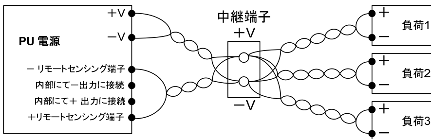
図 2-10 中継端子を用いた複数の負荷への接続
