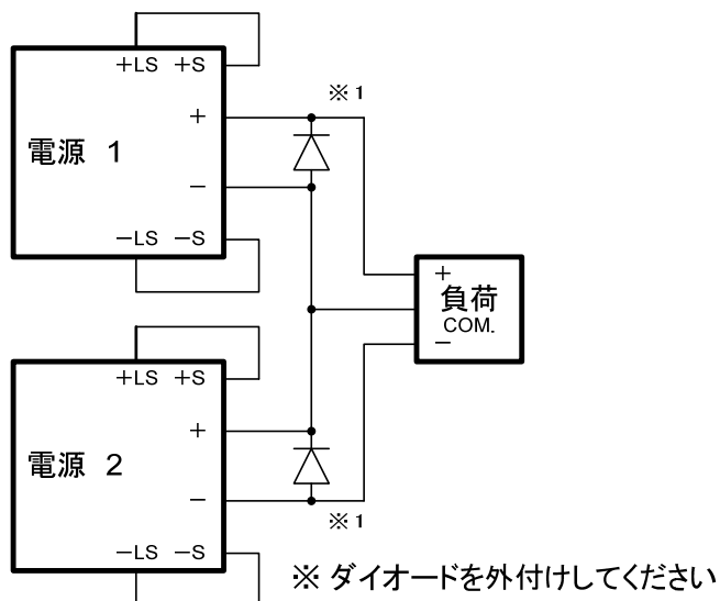
図 4-3 バイポーラ出力電圧用直列接続
