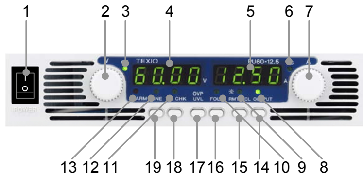
図 3-1 フロントパネル
