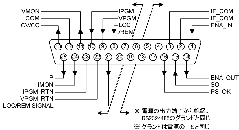
図 3-4 J1 接続端子と機能
