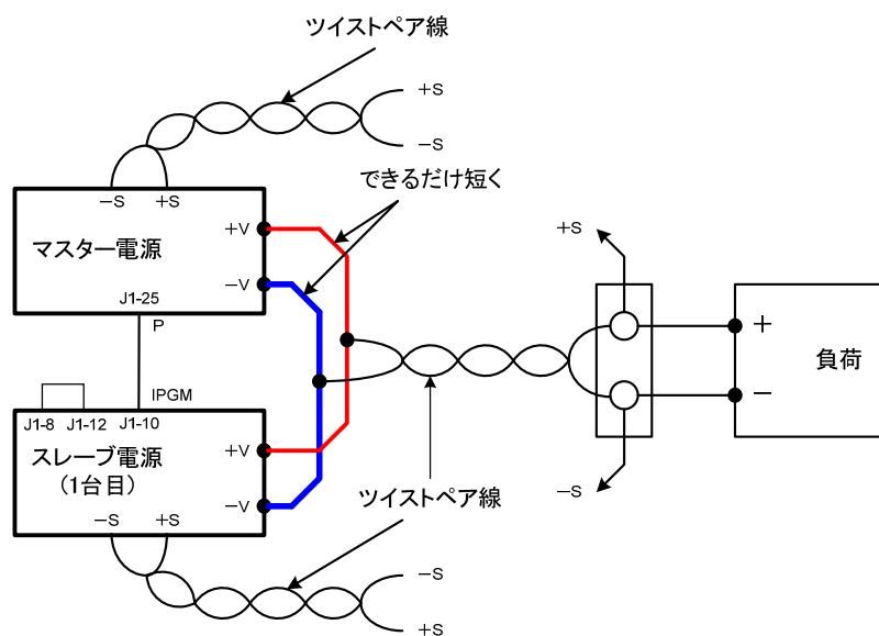
図 4-5 リモートセンシングによるマスタースレーブ並列運転
