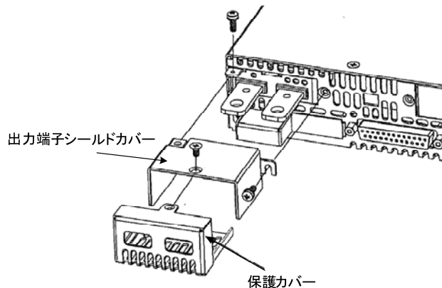
図 2-3 出力端子シールドカバーと保護カバー(60V タイプのみ)の取付け
