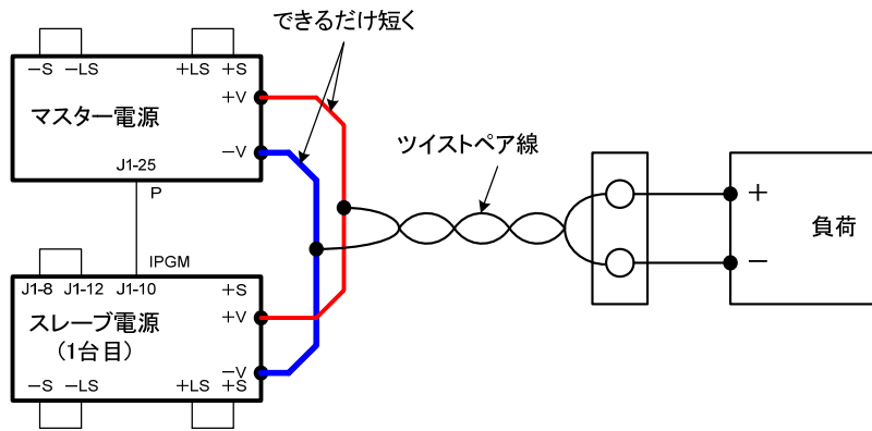
図 4-4 ローカルセンシングによるマスタースレーブ並列運転
