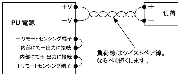
図 2-7 ローカルセンシングによる単一負荷の接続
