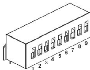
図 3-3 SW1 設定ディップスイッチ
