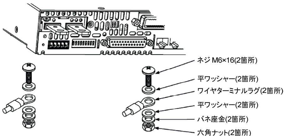
図 2-2 負荷線の接続方法(6V~60V 出力電圧モデル)
