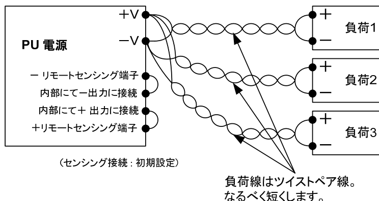
図 2-9 複数の負荷へ接続する場合
